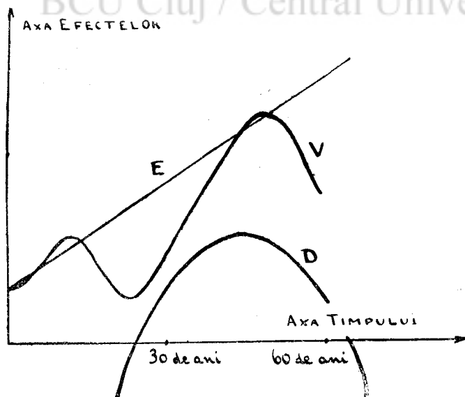
Curbe psihomatematice: V (variația comportamentului normal), E (dreapta de echilibru psihic) și D (parabola de disechilibru). Formulele din text sunt cea mai probabilă interpretare a lor.
