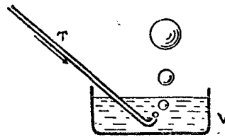
Fig. 31. Formarea bășicilor de săpun pline cu hidrogen.
