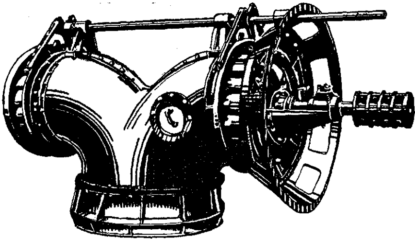
FRANCIS-TURBINE
