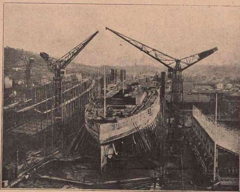
Construirea unui dreadnought, în șantierul dela Toulon cu tot aranjamentul, ce se recere la construirea unui vapor de acesta uriaș. Azi toate statele fac sforțări îngrozitoare, ca să se 'ntreacă în mărirea și întărirea flotelor de războiu, și asta — pentru ca să asigure pacea.
